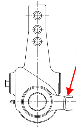
オートマチックスラックアジャスタのコントロールアーム (対策品)
