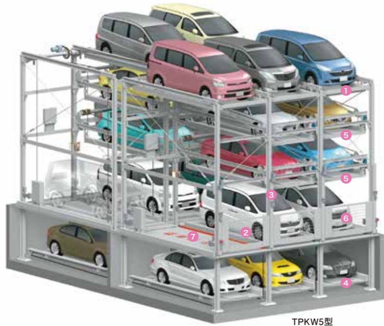
機種ラインナップ (地上3段仕様もございます)
