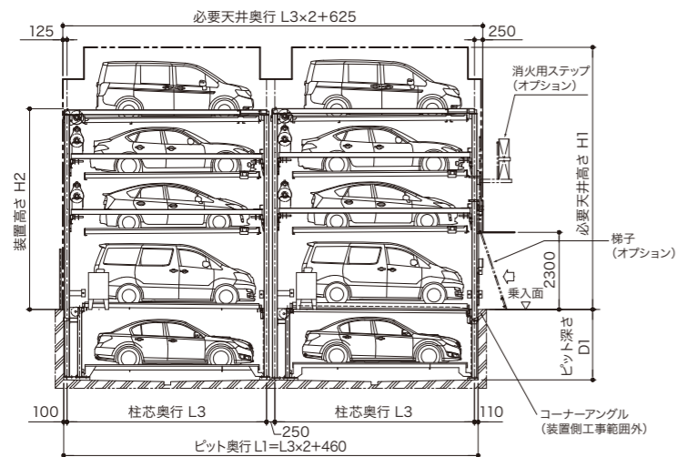
側面図 (一体型)
