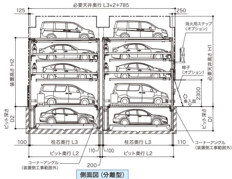
側面図 (分離型)
