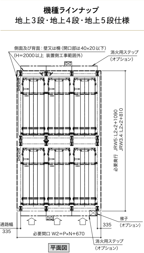
平面図
