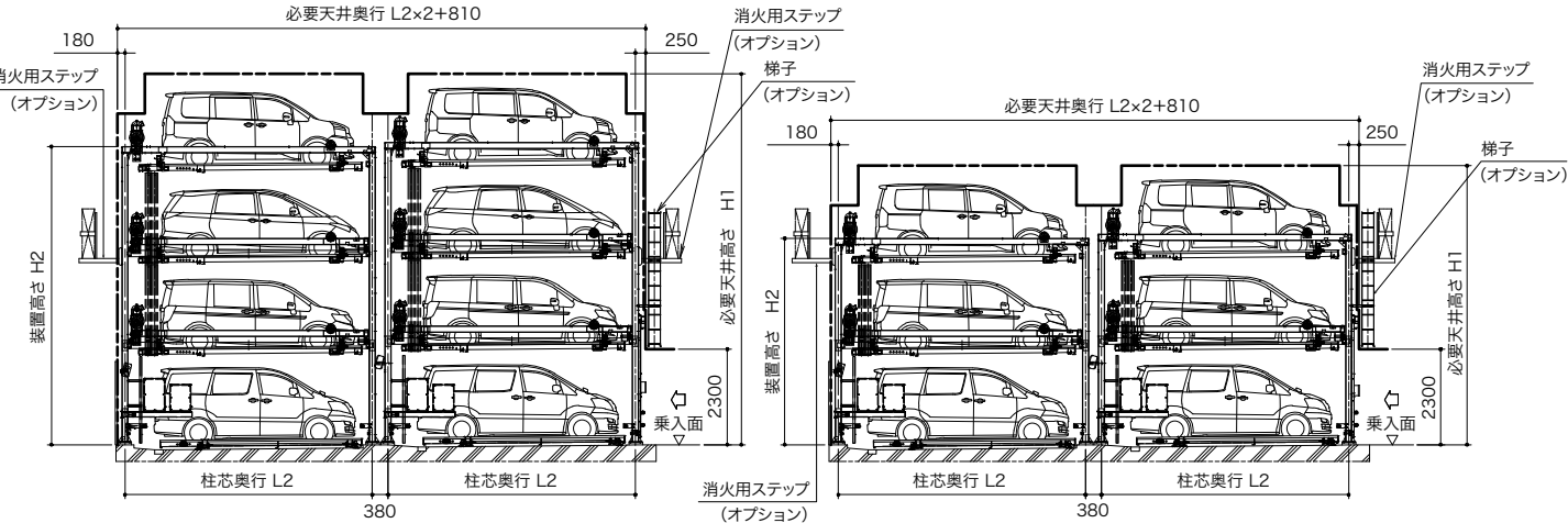
TPJRW4型 側面図
