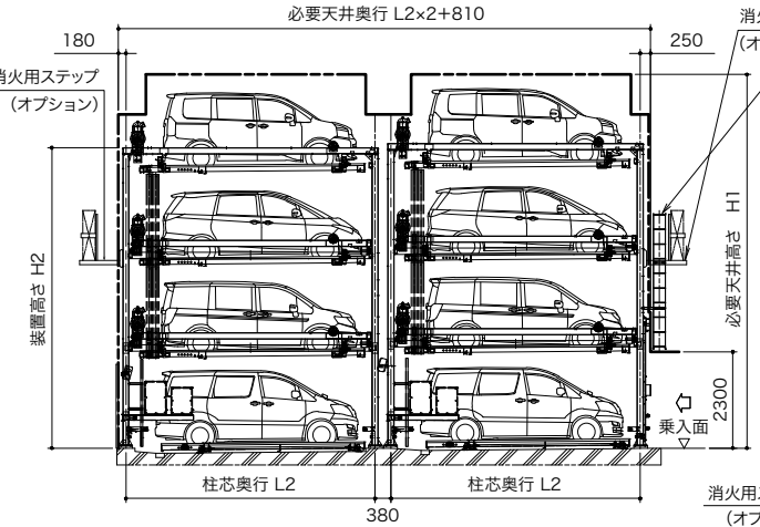
TPJRW4型 側面図
