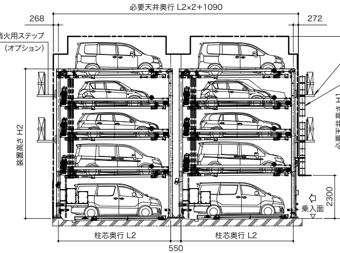
TPJRW5型 側面図
