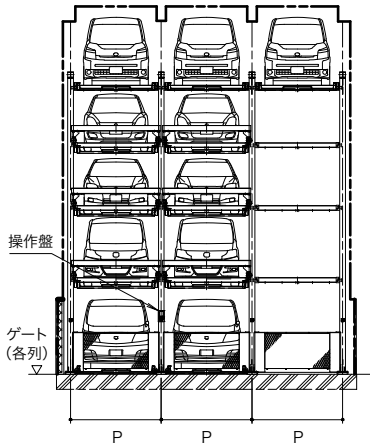
正面図
