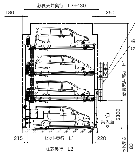
側面図
