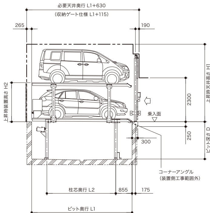
側面図
