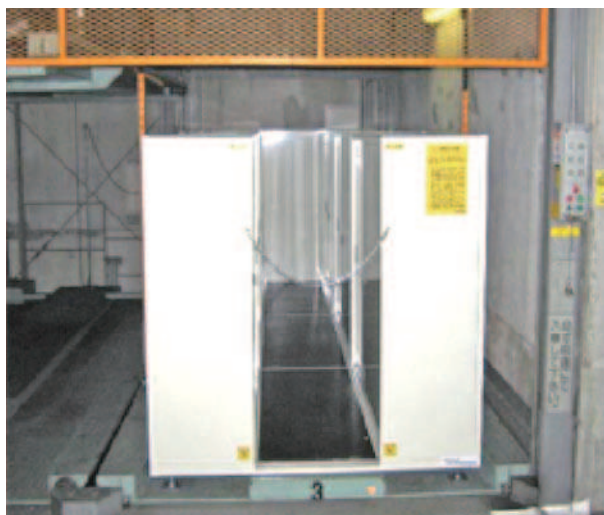
搬器上に倉庫を設置した例
