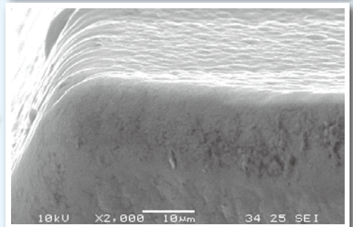
ダイヤモンドコート表面 / Diamond coating surface conditions
