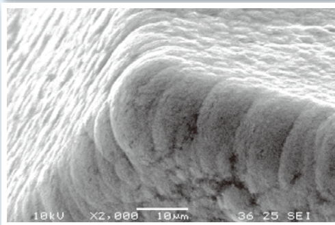
ダイヤモンドコート表面 / Diamond coating surface conditions
